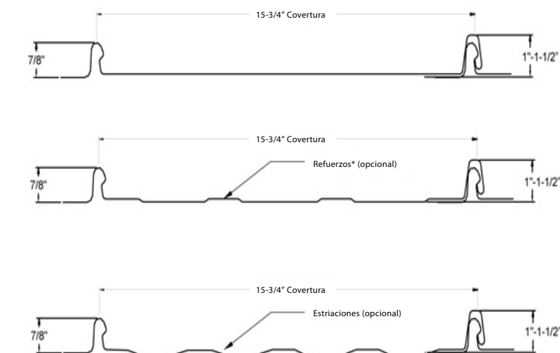
US-150NS Perfil del Standing Seam Panel
